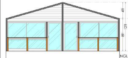
ELEVATION-A
