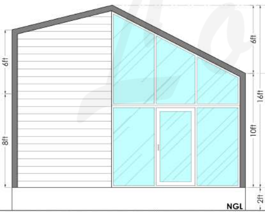
ELEVATION-A
