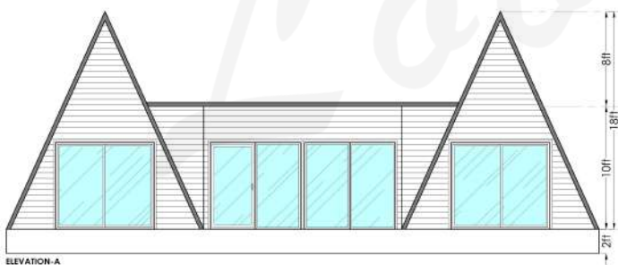
ELEVATION-A
