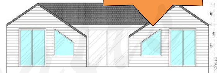
ELEVATION-A
