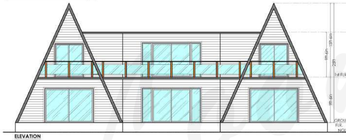
ELEVATION-A
